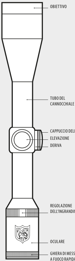
REGOLAZIONE DELLA PARALLASSE
